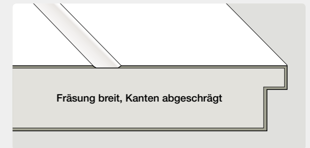
Querschnitt | Lines STRAIGHT
